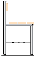
dress-6250 - Bankkonsole mit Gleitfüßen oder Bodenbefestigung, integrierter Rückenlehne, Schuhrost optional
